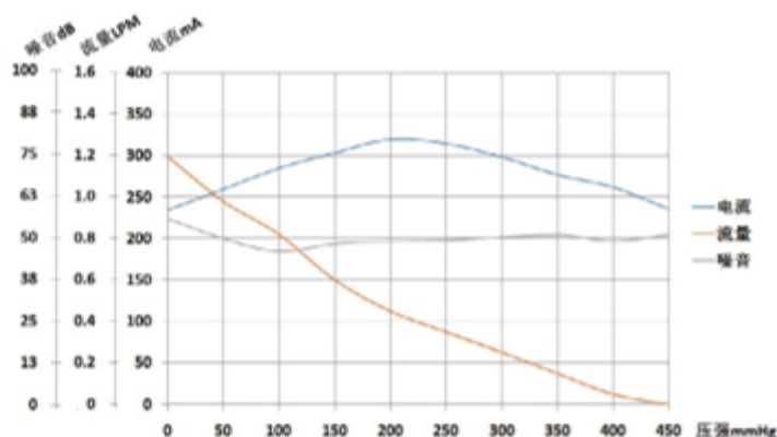
WP12-3特性曲线图
