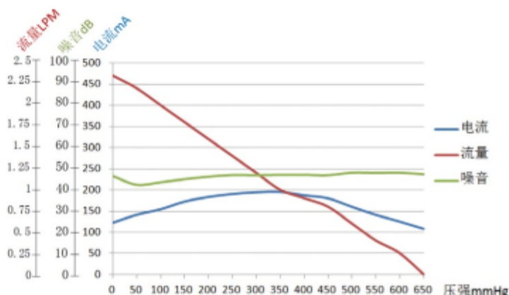
WP27D-12特性曲线图
