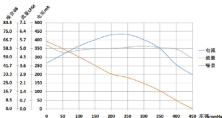
WP32B-12特性曲线图
