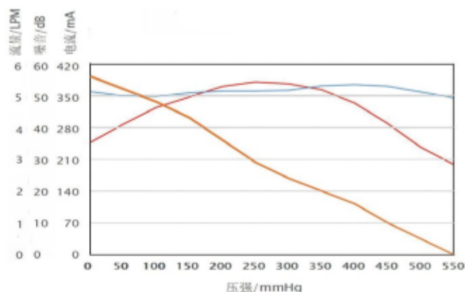
WP32E-12特性曲线图
