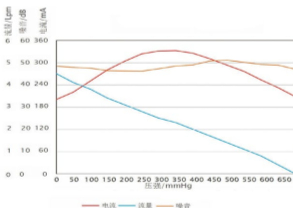
WP32F-12特性曲线图
