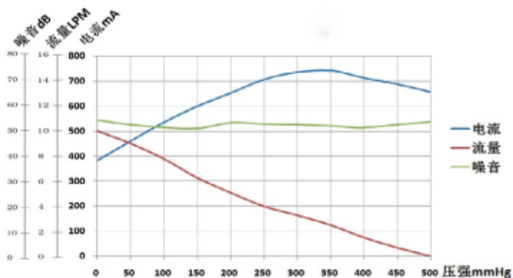
WP40-12特性曲线图
