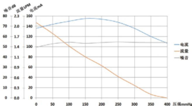
WPV27C-12特性曲线图
