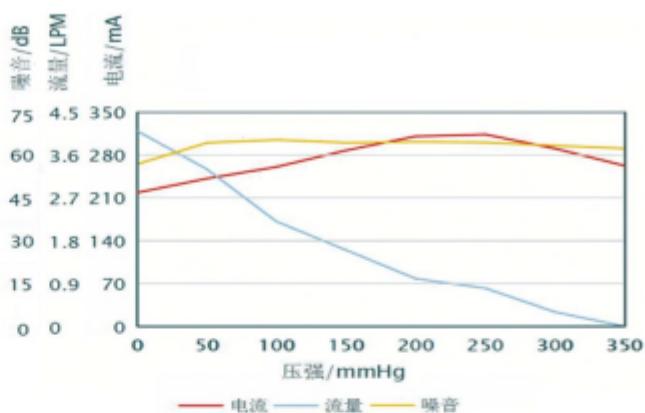
WPV32F-12特性曲线图
