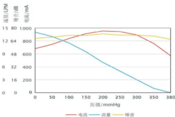
WPV36-12特性曲线图
